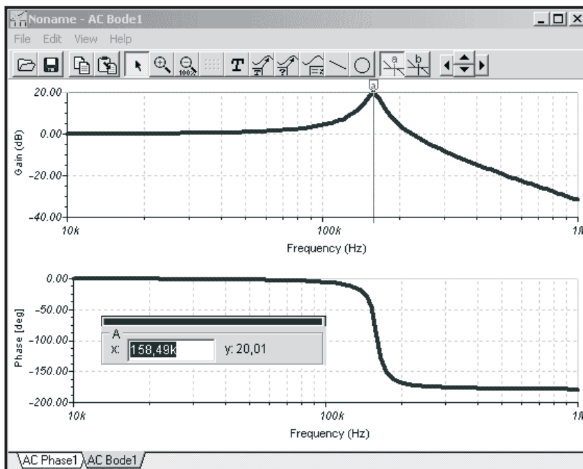
Figuur 60: Het Bode-diagram geeft het amplitude- en faseverloop in functie van de frequentie van het ingangssignaal.
