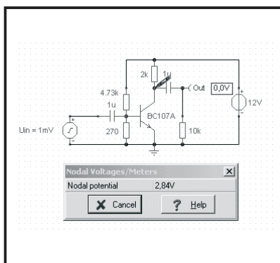
Figuur 10: De meest eenvoudige analyse is deze “DC Node Voltage”, waarmee u de gelijkspanning op alle punten van uw schema kunt meten.
