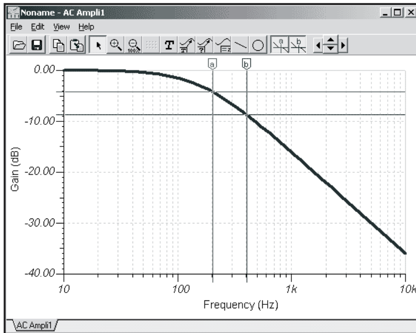
Figuur 42: De amplitude/frequentie-grafiek van de schakeling van figuur 41.
