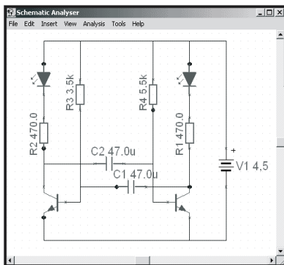
Figuur 3: In het venster van de “Schematic Analyser” ziet u het schema van uw schakeling onderdeel na onderdeel groeien.
