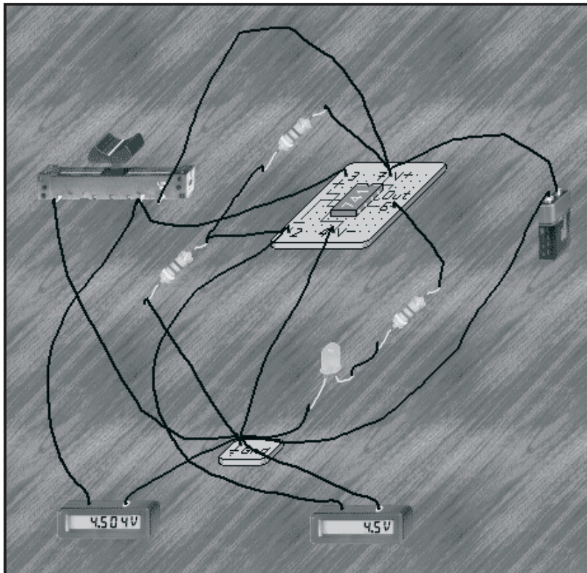
Figuur 29: Het toevoegen van twee voltmeters die bewijzen dat de uitgang omklapt als de spanningen op de twee ingangen van de op-amp aan elkaar gelijk zijn.
