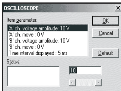
Figuur 35: Het instellingenvenster voor de oscilloscoop.
