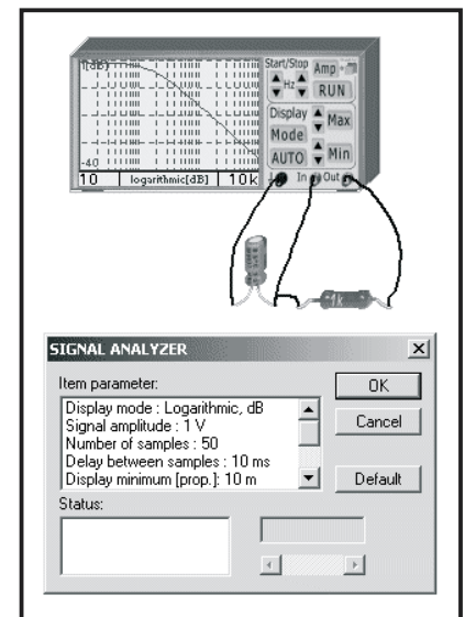
Figuur 41: Het gebruik van de frequentie-analyser bij het opmeten van weergavekarakteristiek.
