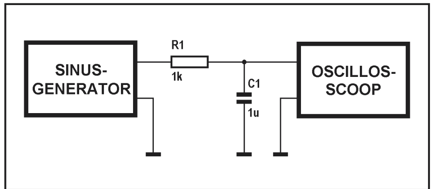
Figuur 40: Een RC-kring vormt een laagdoorlaat filter.
