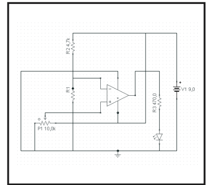
Figuur 28: Het geoptimaliseerde schema van uw comparatorschakeling.
