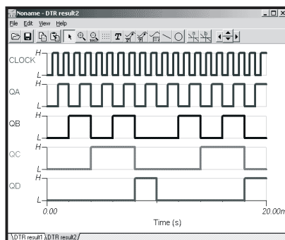
Figuur 65: De digitale tijd analyse van de tienteller.
